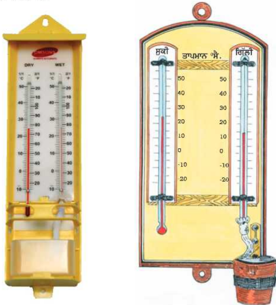
ਚਿੱਤਰ 3.3 ਉੱਚਤਮ ਤੇ ਨਿਊਨਤਮ ਥਰਮਾਮੀਟਰ
