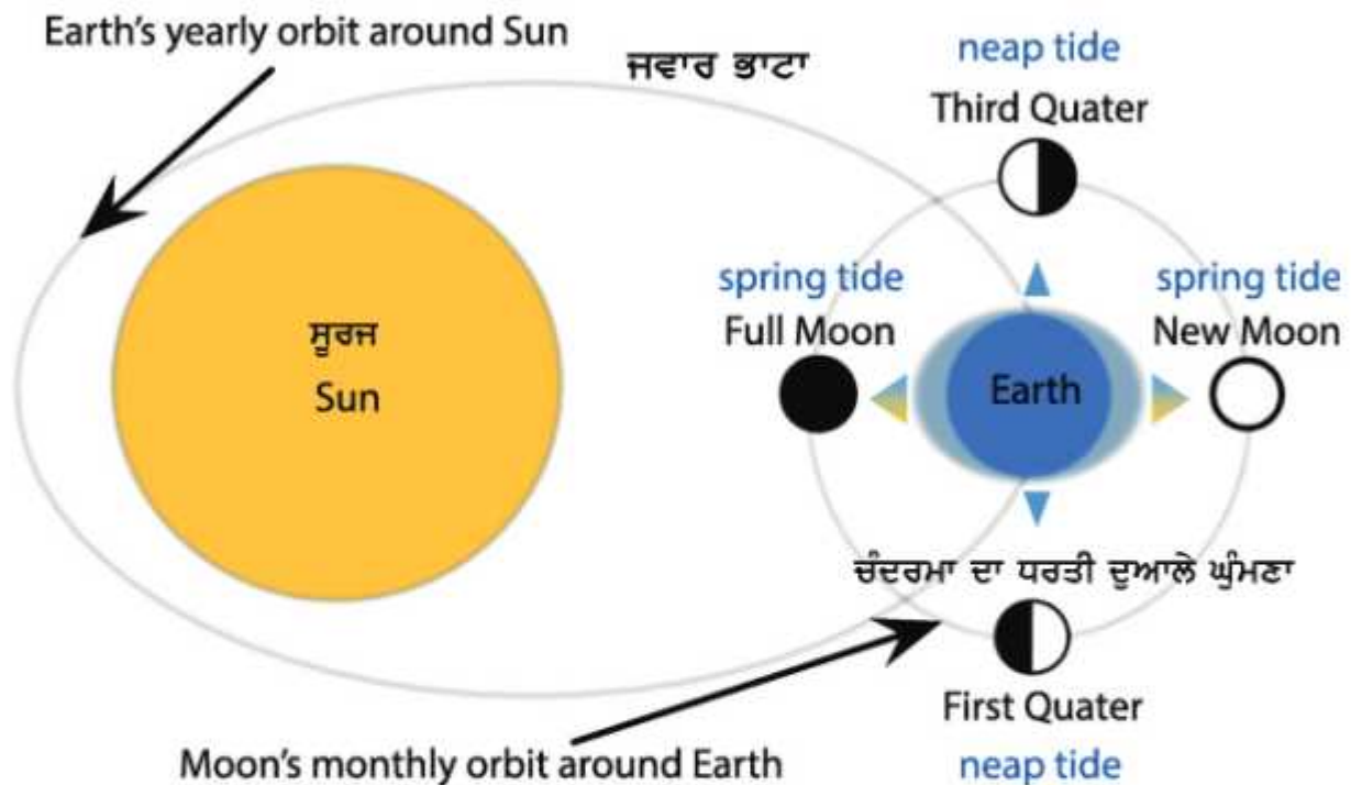
ਚਿੱਤਰ 4.8 ਛੋਟਾ ਜਵਾਰਭਾਟਾ
