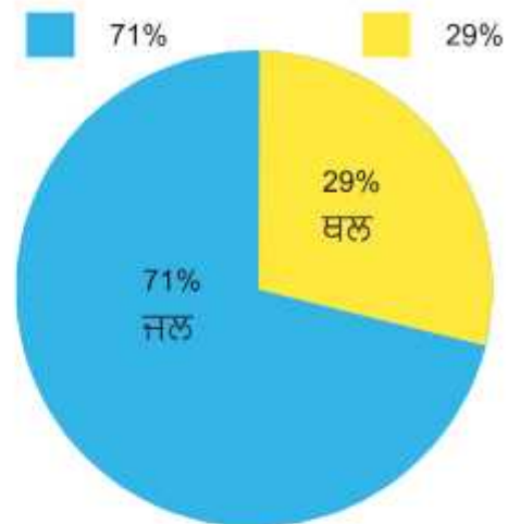
ਚਿੱਤਰ 1.2 ਧਰਤੀ ਤੇ ਜਲ ਅਤੇ ਥਲ ਦੀ ਵੰਡ
