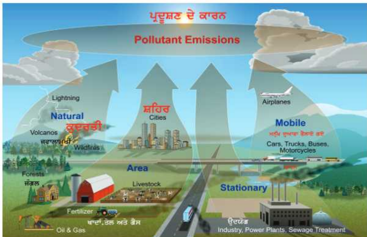
ਚਿੱਤਰ 3.1 ਹਵਾ ਪ੍ਰਦੂਸ਼ਣ
